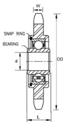
# 40-60 Sprockets
